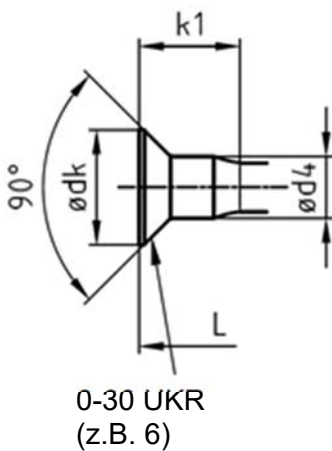
Kopf "K" Senkkopf mit Bund
