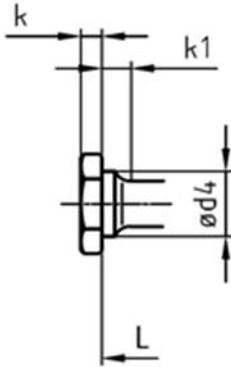
Kopf "J" Dualkopf mit Bund
