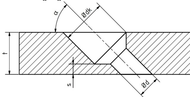
Werden Schmid Schrauben mit Senkkopf geneigt in Bauteile aus Metall eingebracht, sind die Bohrungen unter einem Winkel 30^\circ \leq \alpha < 90^\circ zur Achse des Metallbauteils größer auszuführen als der Gewindeaußendurchmesser d und Kopfdurchmesser d_k der Schraube. Die Dicke s unter der konischen Kopfeinsenkung muss zudem die in Abbildung A6.3 angeführten Randbedingungen erfüllen.
