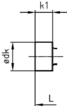
Kopf "L" Zylinderkopf
