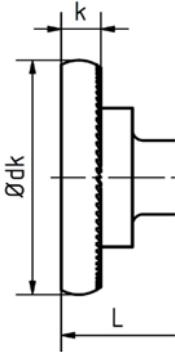
Kopf "G2" Stufenkopf mit Sägezahn
