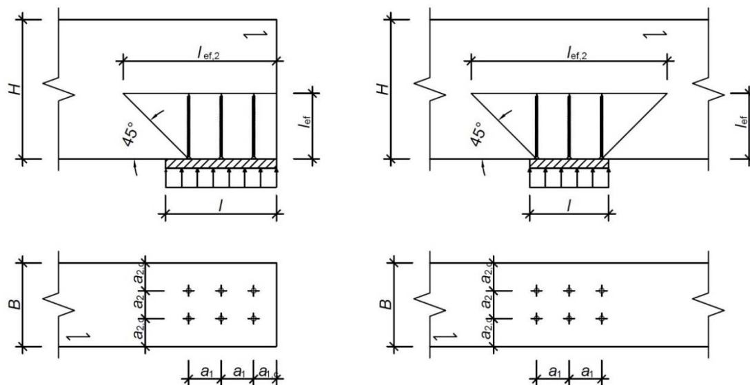
Abbildung A8.1: Querdrukverstärkung von Holzbauteilen: Endauflager (links) Mittelaufleger (rechts)
