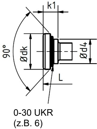
Kopf "L" Zylinderkopf
