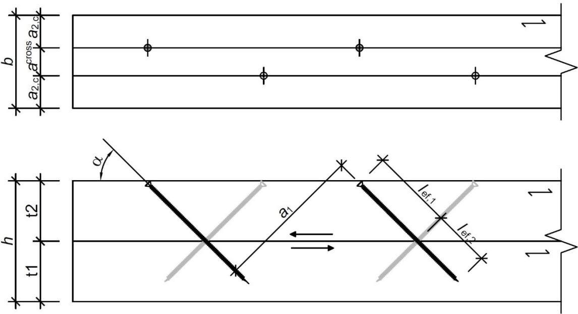
Abbildung A7.2: Beispiel für nachgiebig verbundenen Biegeträger oder Rippendecke
