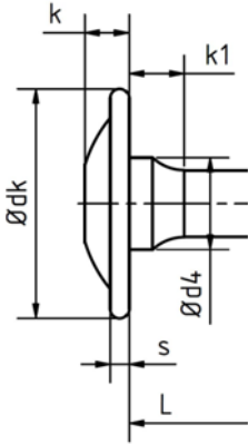
Kopf "G1" kleiner Scheibenkopf mit Bund
