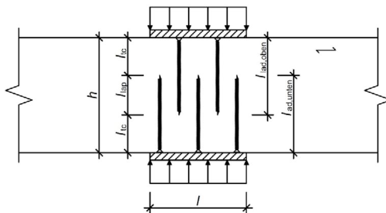
Abbildung A8.2: Querdrukverstärkung von Holzbauteilen mit Schmid Schrauben bei einer Lastdurchleitung
